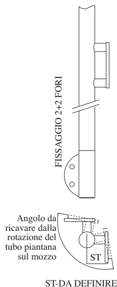
PIANTANA D'ANGOLO O DI TESTATA DOPPIA SEMIROSETTA- MOZZO GIREVOLE
