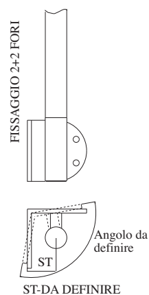
PIANTANA D'ANGOLO-ROSETTA SAGOMATA-MOZZO GIREVOLE
