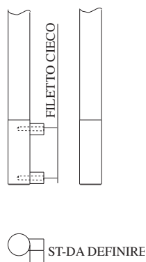
PIANTANA SENZA ROSETTA MOZZO GIREVOLE FILETTATO CIECO
