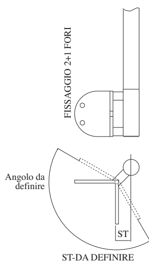
PIANTANA D'ANGOLO ROSETTA SAGOMATA- MOZZO GIREVOLE
