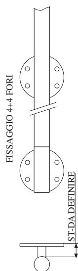
PIANTANA PROLUNGATA CON DOPPIA ROSETTA- MOZZO GIREVOLE
