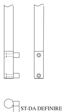
PIANTANA SENZA ROSETTA MOZZO GIREVOLE FORATO PER VITI TCEI
